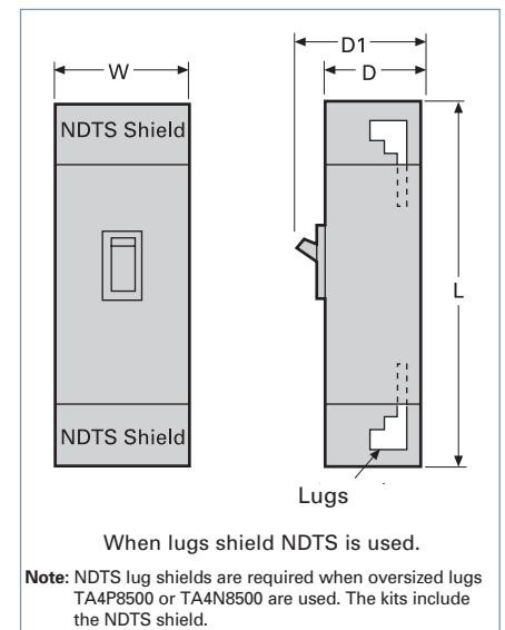
NXD63B120
